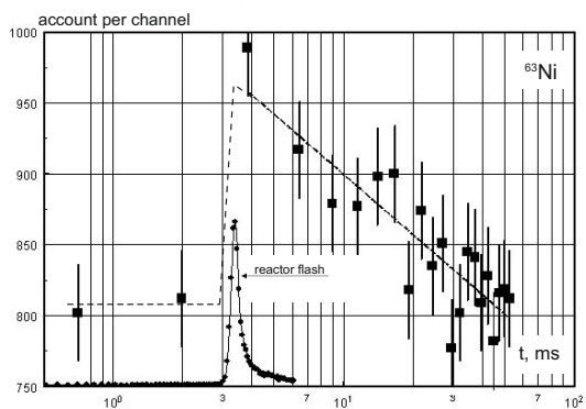
Рис. 25: Результат накопления зарегистрированных бета-электронов, излученных источником ^{63}\text{Ni} .
